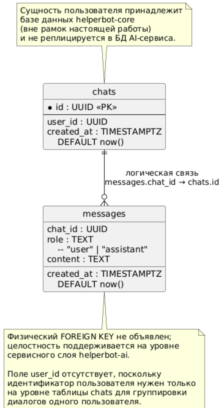
Рисунок 1.4 – ER-диаграмма базы данных helperbot-ai
