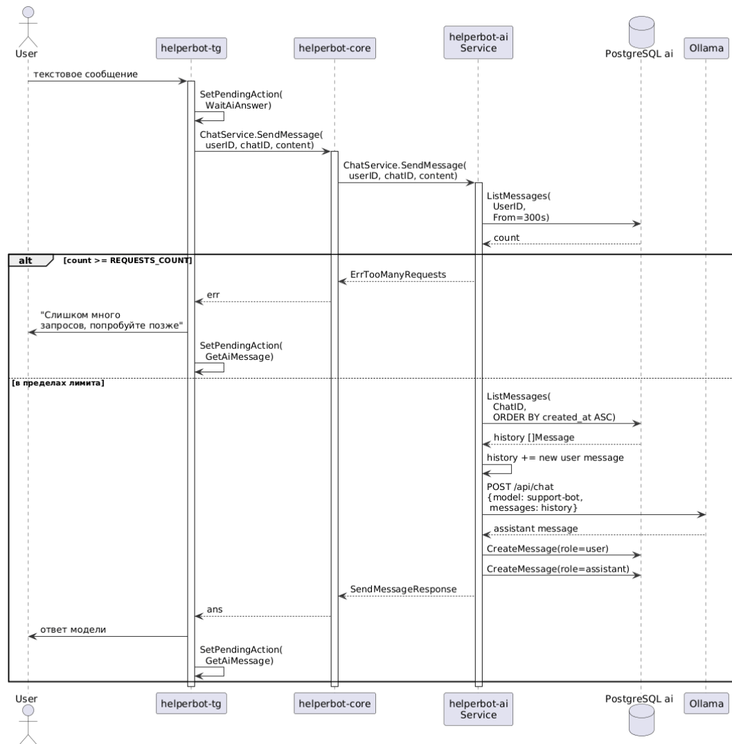
Рисунок 1.3 – Диаграмма последовательности SendMessage
